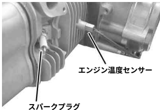
スパークプラグ
