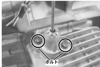
ファンカウリング
