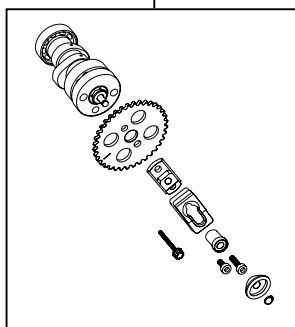
01-08-0164 カムシャフト (S-20D オートデコンプ)
