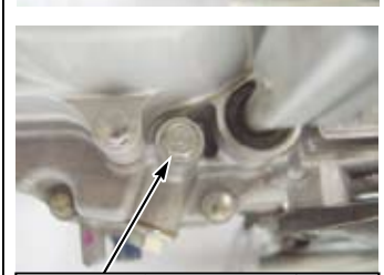
オイルフィラボルト / シーリングワッシャ
