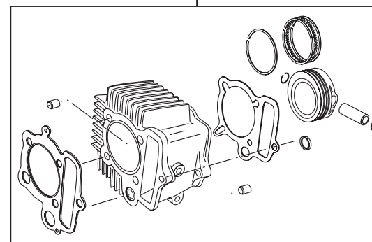
01-04-7004 シリンダーキット 106cc(スカットシリンダー)
