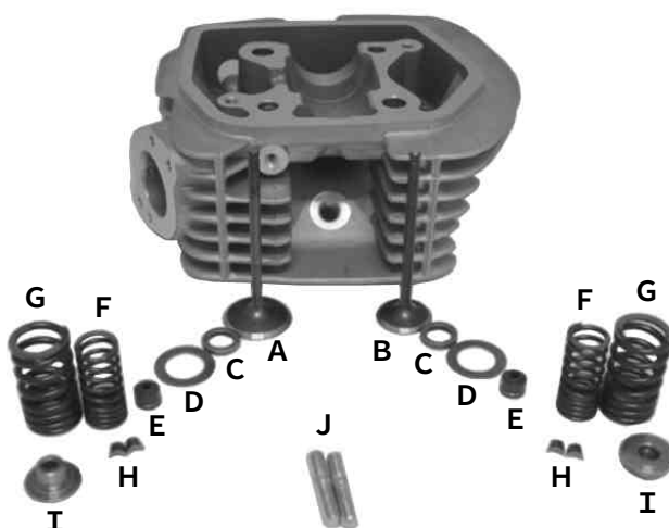
シリンダーヘッドインナーパーツ
