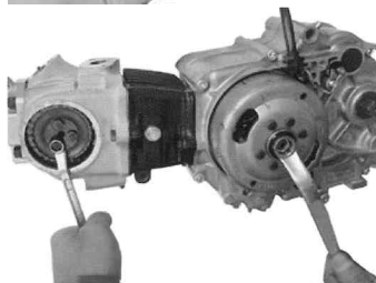
バルブクリアランス (インテーク側)
