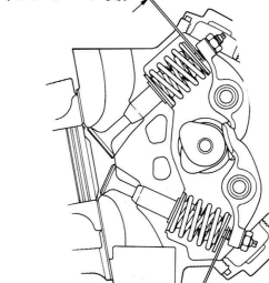
バルブクリアランス (エキゾースト側)
