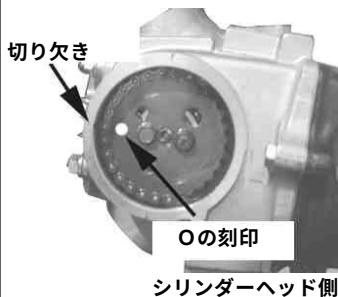
シリンダーヘッド側
