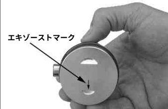
◇ピストンヘッド部三角マークの先を下（エキゾースト側）になるようにしてピストンを取り付ける。
