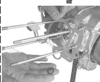
Oリング
