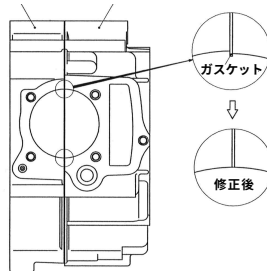
スリーブ 干渉部分
