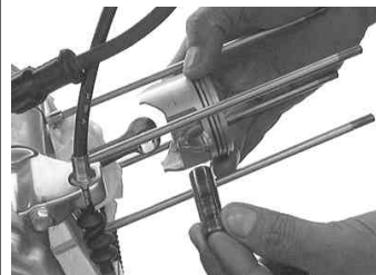
◇ピストンに三分の一程度ピストンピンを挿入しておいて取り付けるのも簡単な方法ではある。 ◇付属のピストンピンサークリップをサークリップ溝にきっちりとはめ込む。
