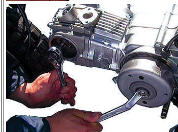
バルブクリアランス (エキゾースト側)
