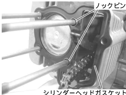
シリンダーヘッドガスケット
