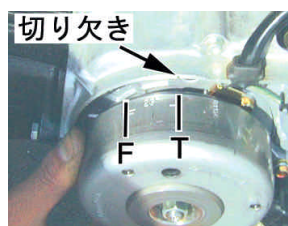
フライホイール側
