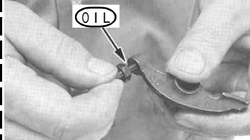
キット内のロッカーアーム、アジャストボルトにエンジンオイルを塗布します。
