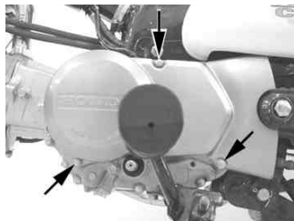
クランクケース左カバーを止めているボルト3本を取り付ける。 使用工具 8mmボックスレンチ&ショートジョイント 締め付けトルク 10 N・m (1.0 kgf・m)
