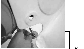
クランクケース左カバーを止めているボルト3本を取り付ける。 使用工具 8mmボックスレンチ&ショートジョイント 締め付けトルク 10 N・m (1.0 kgf・m)
