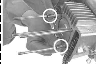
シリンダーヘッド面とシリンダー上面をシンナー等で脱脂する。
