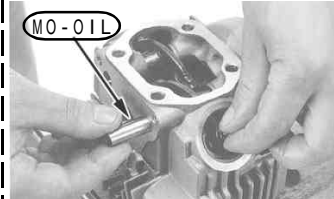
オリジナルのロッカーアームシャフトにモリブデン溶液を塗布し、ロッカーアームシャフトのネジ部を外側に向け、ロッカーアームとストッパープレートの穴位置を合わせ、ロッカーアームシャフトを取り付けます。
