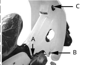
A部に12mmのふくろナットをレッグシールドとの間にプレートをはんで締め付ける。B部に10mmの長ボルトをレッグシールドの裏にスペーサーをはんで締め付ける。C部に10mmのボルトをワッシャをはんで締め付ける。左側も同様に取り付け。
