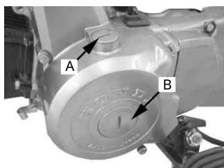
セル付の場合は、A、Bの2つを取り付け、締め付けます。 使用工具 マイナスドライバー 締め付けトルク A 2 N・m (0.2 kgf・m) B 3 N・m (0.3 kgf・m)
