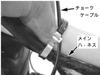
チョークケーブルとメインハーネスをバンドで束ねます。
