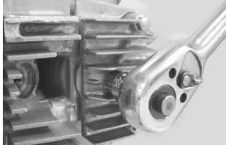
シリンダーヘッド右側の6角ボルト(矢印)を締める。 使用工具 10mmボックスレンチ 締め付けトルク 12 N・m (1.2 kgf・m)
