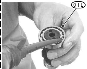
専用のカムシャフトの両端のベアリングにエンジンオイルを塗布します。
