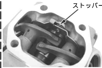
シリンダーヘッドにキット内のストッパープレートのストッパー部をシリンダーヘッド右側に向け、ロッカーアームと共にセットします。
