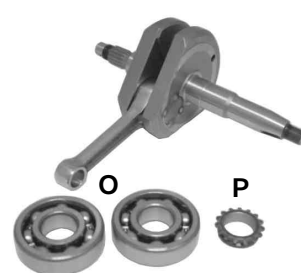
クランクシャフトリペア
