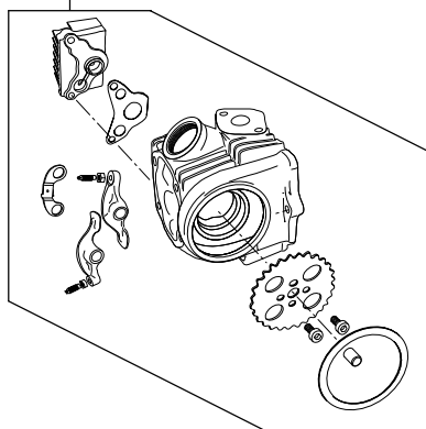
01-08-0015D カムシャフトR-15
