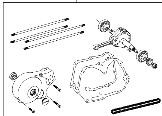
01-10-8042T ストロークアップクランクキット(54ストローク)
