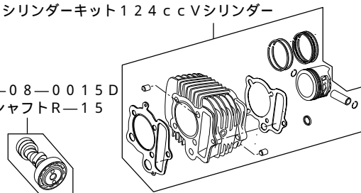
01-04-7124V シリンダーキット124cc Vシリンダー
