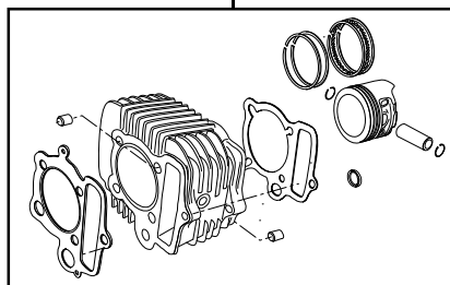
01 04 7124V シリンダーキット124cc Vシリンダー
