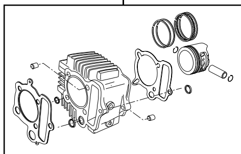
01-04-8106 シリンダーキット106ccシリンダー
