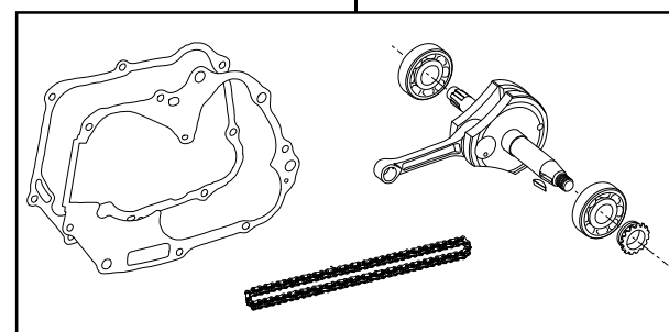
01-10-8432 ストロークアップクランクキット (50ストローク)
