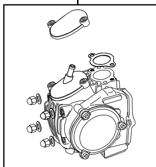
01-03-8004 スーパーヘッド+Rキット
