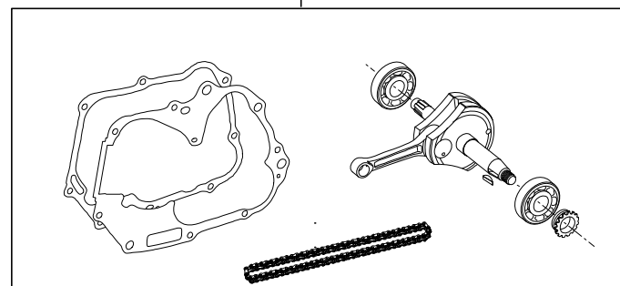
01-10-8432 ストロークアップクランクキット（50ストローク）
