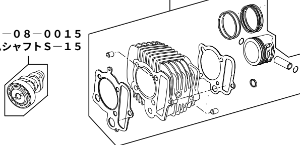
01-04-8106VA シリンダーキット106ccメッキVシリンダー
