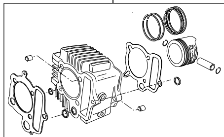
01-04-8106 シリンダーキット124ccシリンダー
