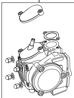
01-03-8004 スーパーヘッド+Rキット
