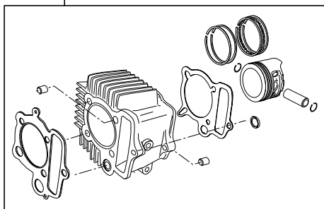
01-04-8106H シリンダーキット106cc Hシリンダー
