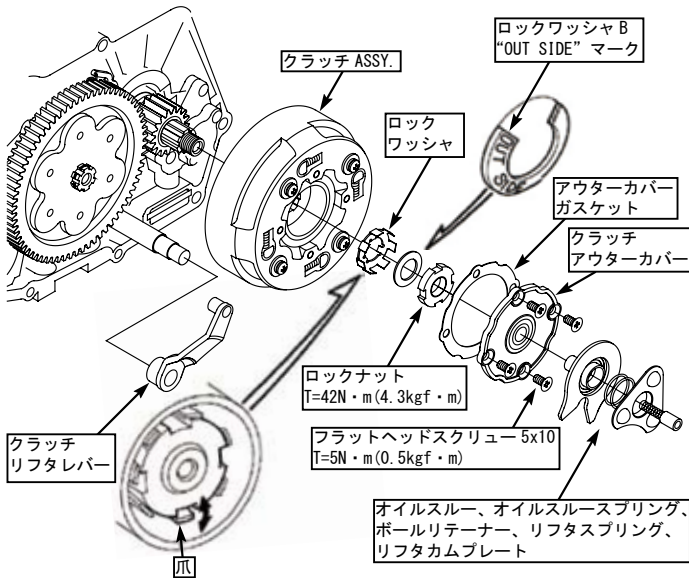
一次側遠心クラッチ
