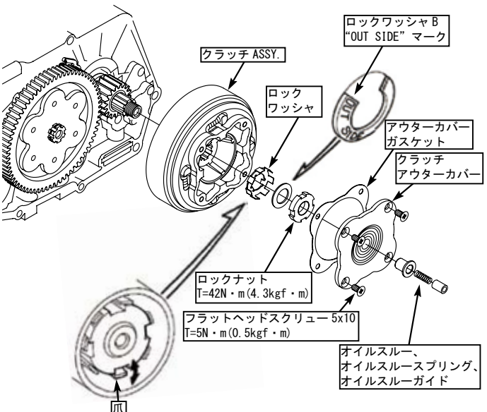
一次側マニュアルクラッチ
