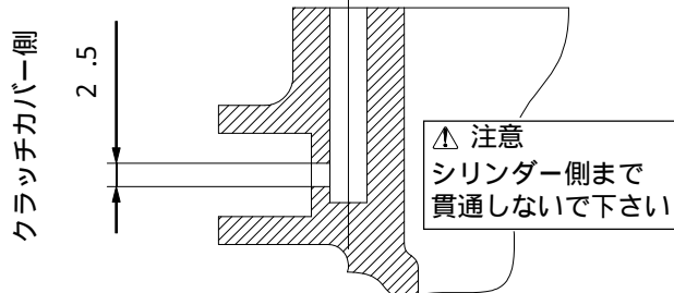
オリフィス部断面図
