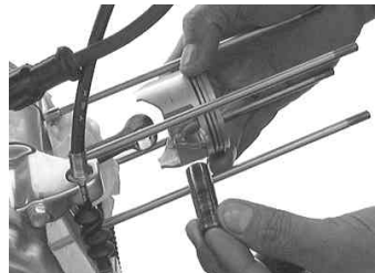
◇ピストンに三分の一程度ピストンピンを挿入しておいて取り付けるのも簡単な方法ではある。 ◇付属のピストンピンサークリップをサークリップ溝にきっちりはめ込む。
