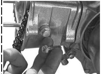
◇シリンダーサイドボルトを取り付ける。（指でしめる程度まで仮止め）
