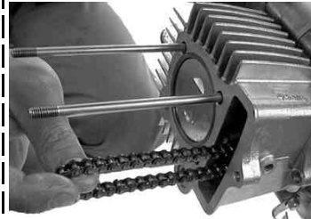
◇カムチェーンを引っ張りながらガイドローラーをつける。
