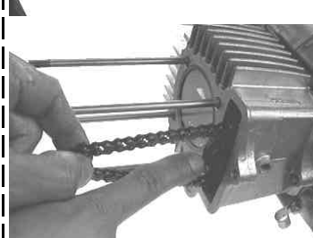
◇シリンダーのガイドローラーボルト穴にガイドローラーのセンターが合う様に押し込む。
