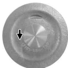
◇ピストン頂点の矢印が下（エキゾースト側）を向くようにピストンを取り付けます。
