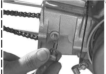
◇ガイドローラーボルトを取り付ける。（指で閉まる程度まで仮止め）
