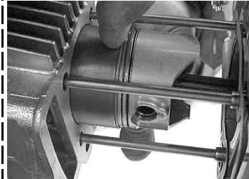
◇シリンダーをピストンリングの合い口がずれないようにしながら指で押し少しづつはめる。ここは難易度が高いです。がんばってください。
