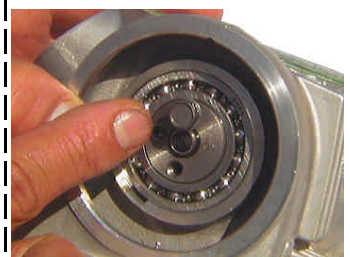
◇カムシャフトにカムスプロケットボルトを取り付け、引っ張るかプラスチックハンマーでヘッドを軽くたたくと抜けてくるので無理に引っ張らずカムシャフトを回しながら取り外す。
