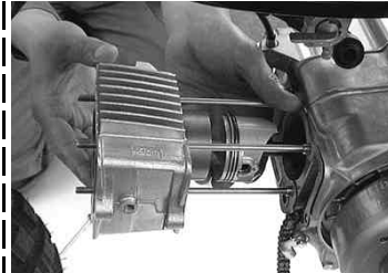
◇タイヤを押さえながらシリンダーを入れていく。
