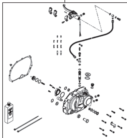
02-01-0161 スペシャルクラッチカバーキット（油圧タイプ）
