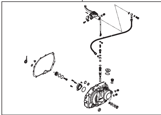
02-01-0167 クラッチカバーキット
