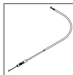
クラッチケーブル COMP. 850mm:00-02-0133
