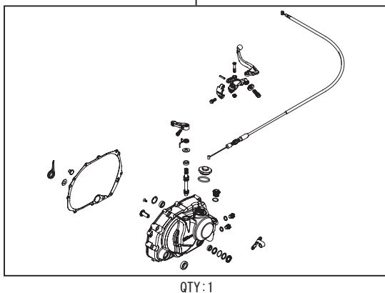
02-01-0357 クラッチカバーキット
