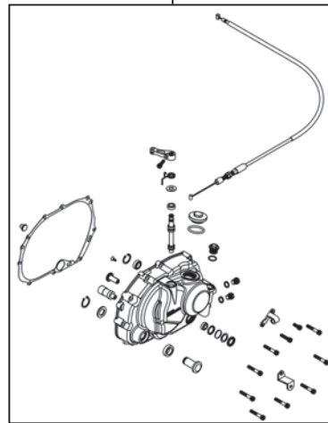
02-01-0153 スペシャルクラッチカバーキット（ワイヤータイプ）
