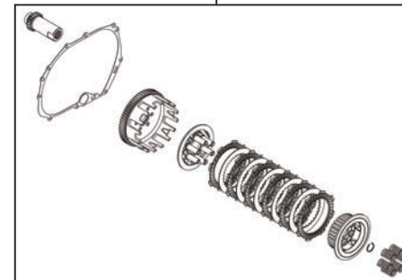
02-01-0330 強化クラッチキット
