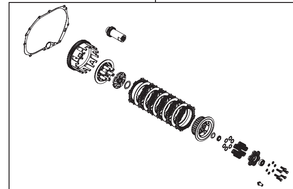
02-01-0171 スペシャルクラッチインナーキット
