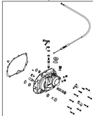
02-01-0153 スペシャルクラッチカバーキット（ワイヤータイプ）
