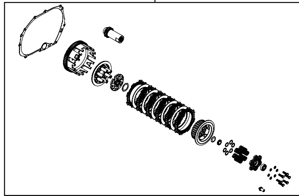
02-01-0171 スペシャルクラッチインナーキット（スリッパ）
