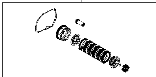
02-01-0330 強化クラッチキット
