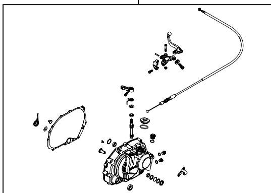
02-01-0405 クラッチカバーキット
