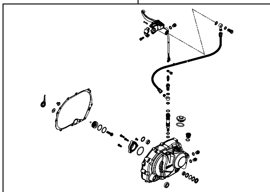
02-01-0407 クラッチカバーキット (油圧)
