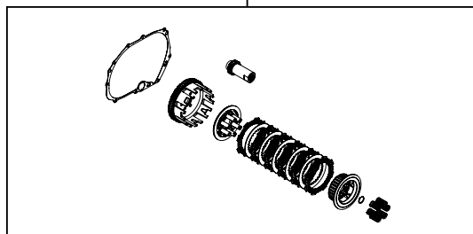
02-01-0330 強化クラッチキット
