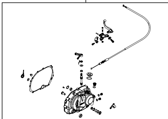
02-01-0409 クラッチカバーキット
