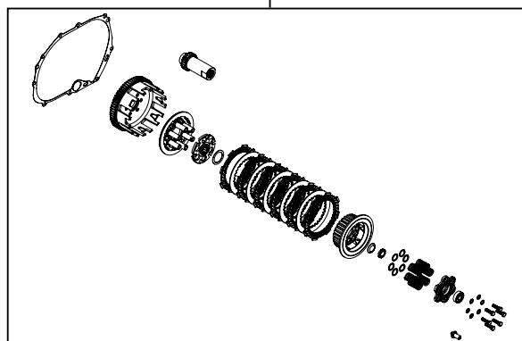
02-01-0171 スペシャルクラッチインナーキット（スリッパ）
