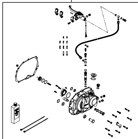
02-01-0413 スペシャルクラッチカバーキット（油圧）
