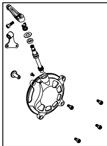
クラッチカバーキット（ワイヤータイプ・乾式） :02-02-0126
