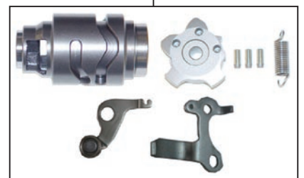
02-04-0294 4速リターンシフトドラムキット
