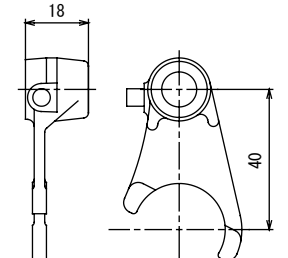
ライトギアシフトフォーク (純正部品)
