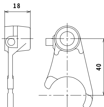
ライトギアシフトフォーク (純正部品)
