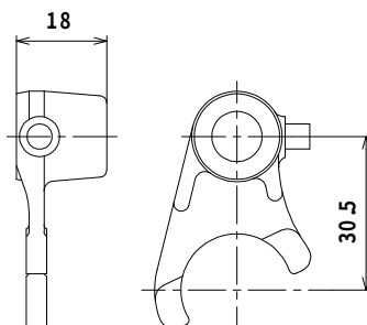
センターギアシフトフォーク
