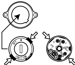
イグニッションスイッチ (正面から見て) イグニッションスイッチ (裏面から見て)
