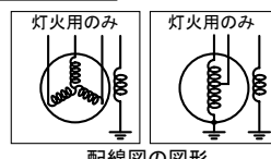
配線図の図形
