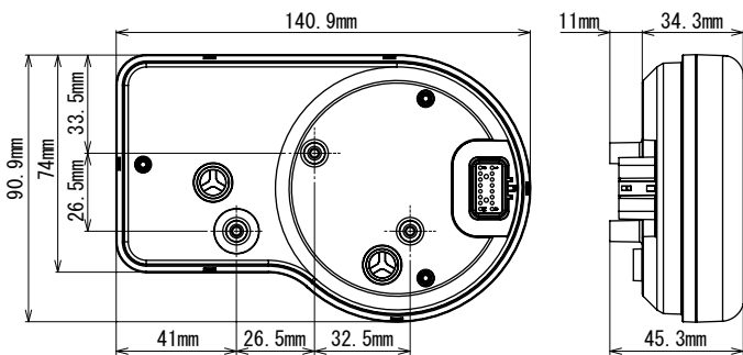
メーター本体寸法図
