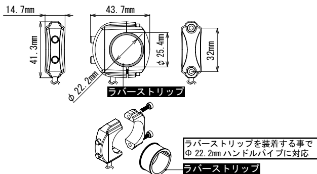
メーター外部スイッチ寸法図
