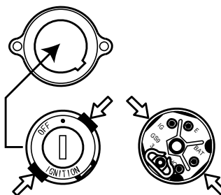
イグニッションスイッチ (正面から見て) イグニッションスイッチ (裏面から見て)
