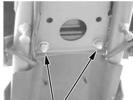
ナットM6 /ワッシャ6mm
