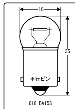
バルブのガラス・口金形状
