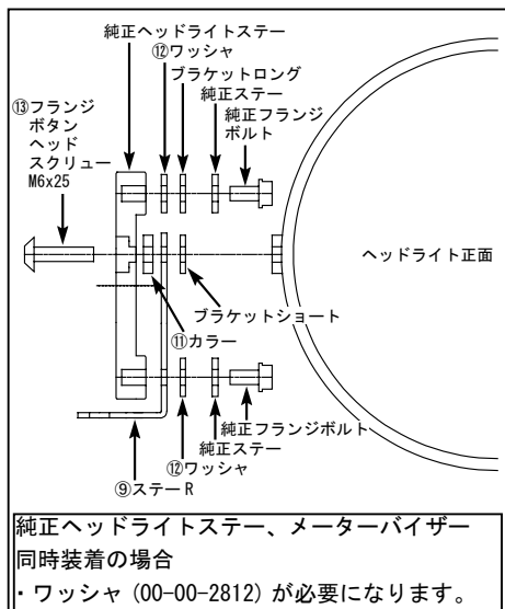
純正ヘッドライトステーの場合
