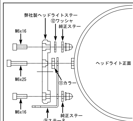
弊社製ヘッドライトステーの場合
