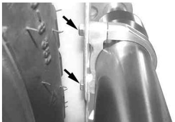
ホイール フロントホイールハブASSY スペーサー
