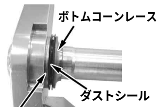
ボトムコーンレース ダストシール ダストシールワッシャ
