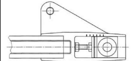
チェーンアジャスター取り付け方向図
