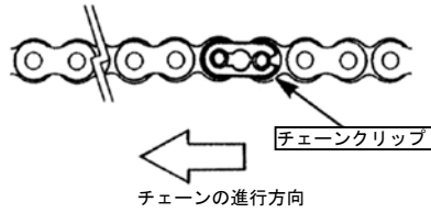
チェーンクリップ チェーンの進行方向
