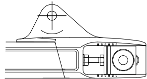
チェーンアジャスター取り付け方向図
